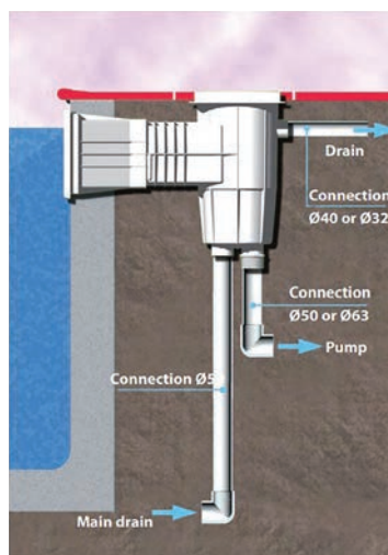
Ugradnja skimera
