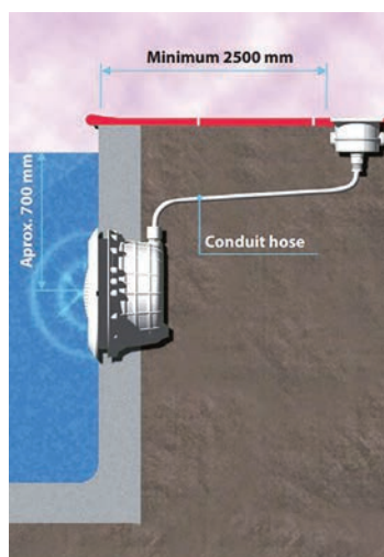
Ugradnja razvodne kutije
