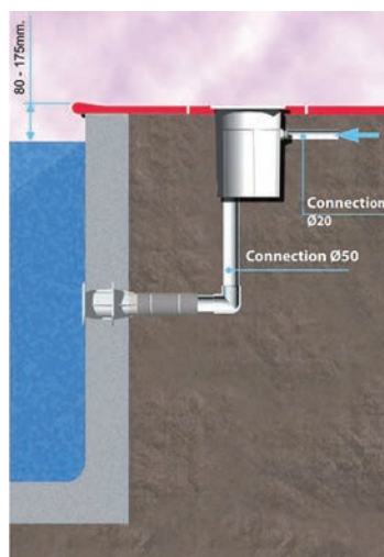
Ugradnja regulatora razine vode
