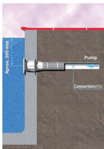
Ugradnja mlaznica
