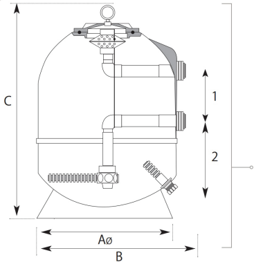
prozirni poklopac
